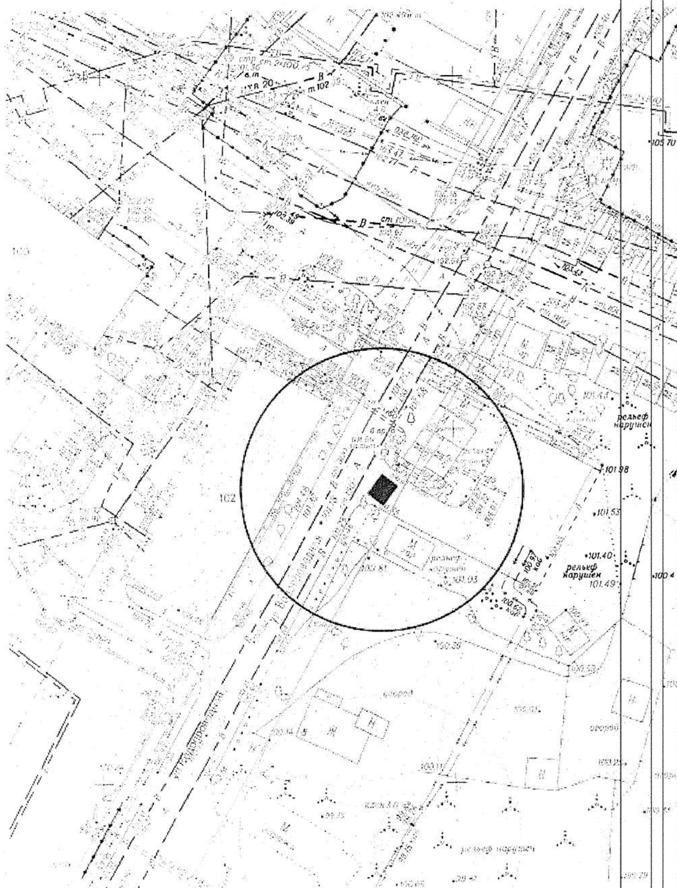
Карта-схема территории №660 по адресному ориентиру улица Обская. (102) на топографическом плане М 1:500
